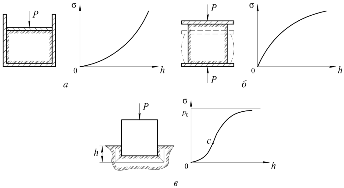
Рис. 2. Сопротивление почвы при деформации: a – компрессионное сжатие; б – сжатие с возможностью бокового расширения; в – вдавливание штампа в массив почвы
