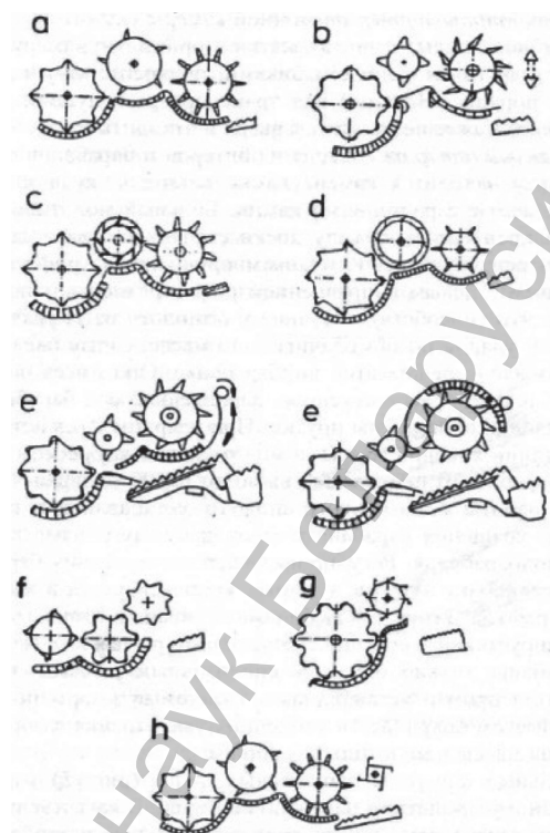
Рис. 2. Конструктивные схемы классических молотильных устройств зерноуборочных комбайнов: а – Ford New Holland; б – Deutz-Fahr; в – MDW, Case IH; д – Dronningbord, Massey Ferguson; е – Fiatagri; ф – Claas; г – John Deere; h – Ford New Holland, Case CF 80
