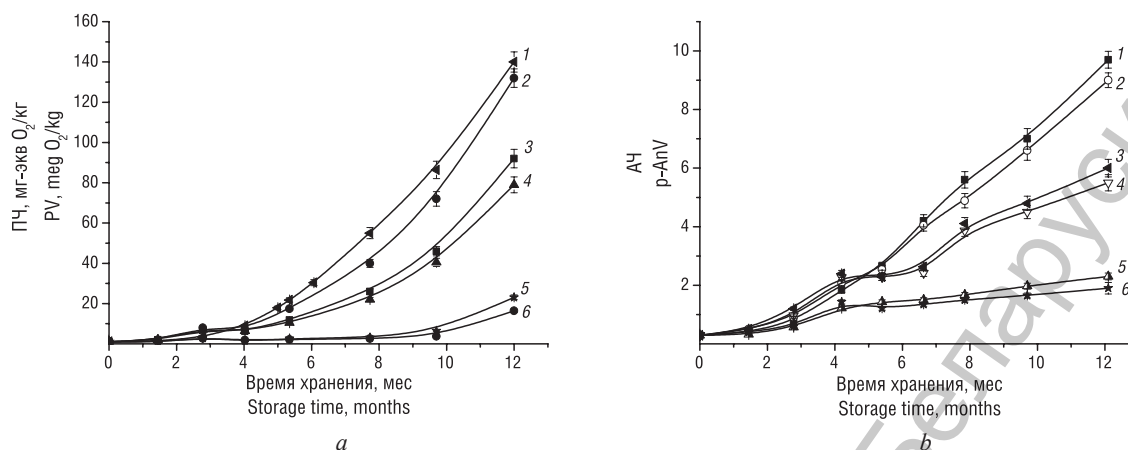
Рис. 5. Накопление гидропероксидов (а) и вторичных продуктов окисления (б) при хранении льняного масла с добавками коэнзима Q 10 и стабилизаторов при комнатной температуре и свободном доступе воздуха: 1 – без добавок; 2 – CoQ 10 , 100 мг%; 3 – CoQ 10 , 100 мг% + СТФ, 1,2 %; 4 – CoQ 10 , 100 мг% + СТС, 1,2 %; 5 – CoQ 10 , 100 мг% + АП, 0,02 %; 6 – CoQ 10 , 100 мг% + СТФ, 1,2 % + АП, 0,02 %
