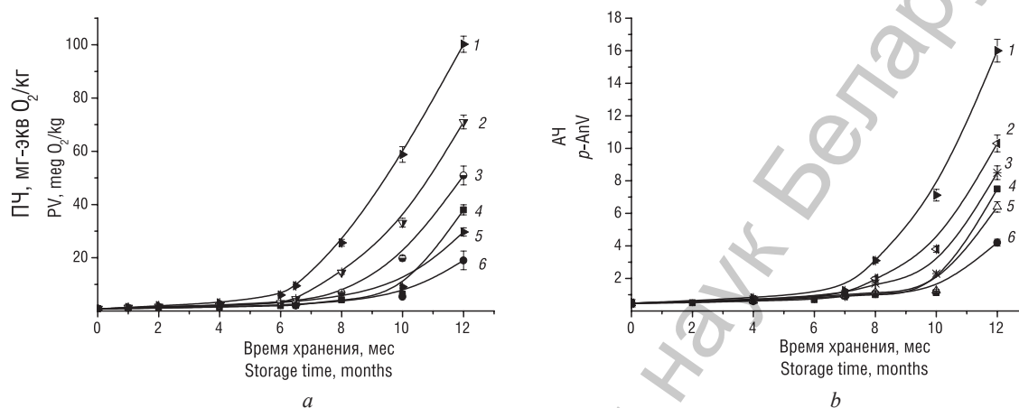
Рис. 2. Изменение пероксидного (а) и анизинового (б) чисел льняного масла с добавками \beta -каротина в процессе хранения при комнатной температуре и свободном доступе воздуха: 1 – Car, 25,0 мг%; 2 – Car, 20,0 мг%; 3 – Car, 15,0 мг%; 4 – масло без добавок; 5 – Car, 10,0 мг%; 6 – Car, 5,0 мг%
