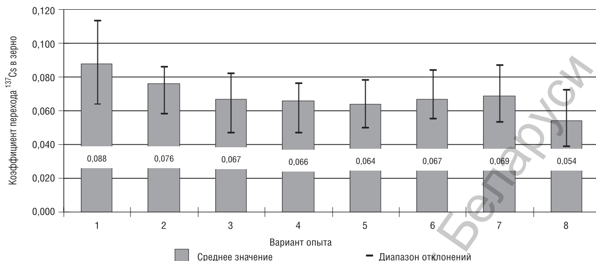
Рис. 1. Коэффициенты перехода ^{137}\text{Cs} в зерно яровой пшеницы в зависимости от доз азотных и калийных удобрений, Бк/кг:кБк/м 2
