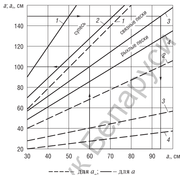
Рис. 4. Глубина вспашки a и слой припахиваемого минерального грунта a_n в зависимости от глубины торфа a_t при соотношении торф:песок в пахотном слое i_1 = 1:2 и в подпахотном профиле i_2 : 1 – 0,5; 2 – 1,0; 3 – 2,0; 4 – 4,0
