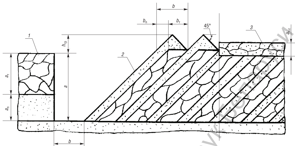
Рис. 2. Технологическая схема глубокой мелиоративной вспашки мелкозалежного торфяника: 1 – почвенный профиль до вспашки; 2 – после глубокой вспашки; 3 – после первичного освоения; a – глубина вспашки; a_t – слой торфа; a_n – слой припахиваемого песка; a_{n.c} – минерально-органический пахотный слой ( a_{n.c} = 20\text{--}25 см); b – ширина захвата плуга; b_t – ширина торфяной прослойки; b_n – ширина песчаной прослойки; h_{гp} – высота гребней
