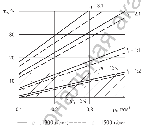
Рис. 3. Влияние соотношения торф : песок i_1 и их плотностей \rho_t и \rho_n на содержание в новом пахотном слое органического вещества m_t
