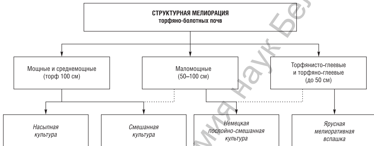
Рис. 1. Схема применения способов улучшения торфяных почв
