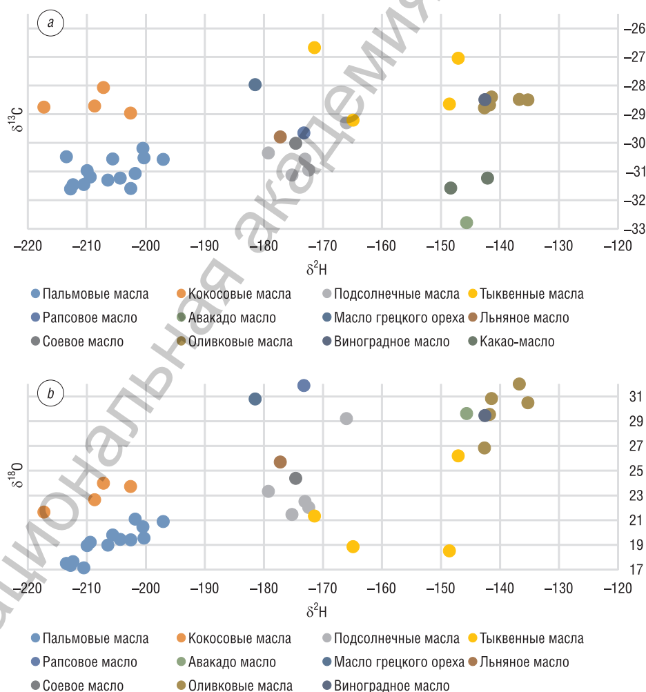
Рис. 4. Изотопный состав растительных масел: a – углерода и водорода; b – кислорода и водорода
