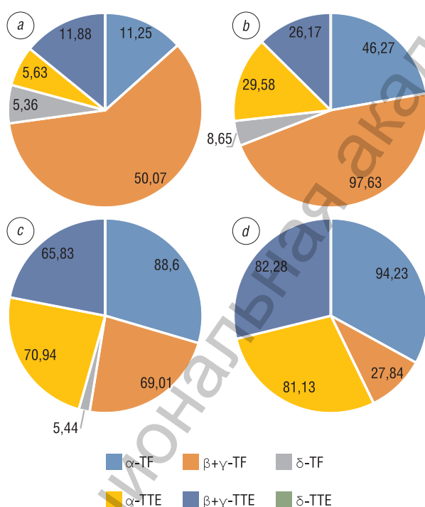
Рис. 3. Токольные составы образцов смеси ПМ+КМ = 10:90 (а), смеси ПМ+КМ = 20:80 (б), смеси ПМ+КМ = 50:50 (с), смеси ПМ+КМ = 80:20 (д), количество токолов указано в [мкг/г]
