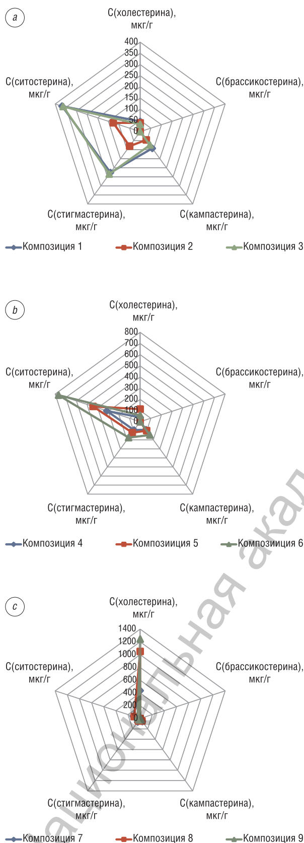
Рис. 2. Диаграмма стеринового состава композиционных смесей: а – I группы; б – II группы; в – III группы
