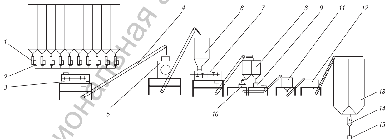
Рис. 2. Технологическая схема лабораторной установки по производству комбикормов для рыб: 1 – весовой дозатор; 2 – задвижка; 3 – смеситель; 4 – конвейер; 5 – дробилка; 6 – бункер перед кондиционером; 7 – кондиционер; 8 – бункеры надгранулятором и надэкструдером; 9 – экструдер; 10 – пресс-гранулятор (комбикорма для карпа); 11 – охладитель-сушилка; 12 – аппарат для вакуумного нанесения жира; 13 – бункеры для готового комбикорма; 14 – весы; 15 – упаковочный аппарат
