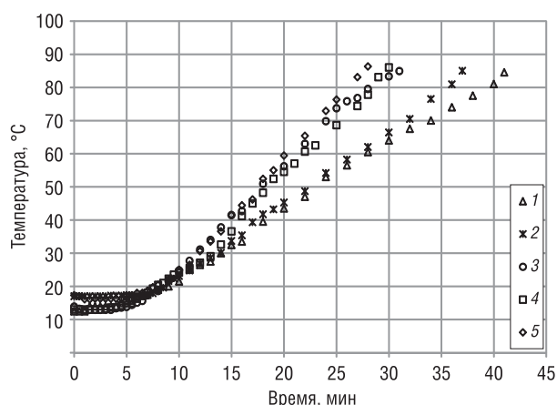
Рис. 2. Изменение температурного поля центра изделий из мясного фарша при температуре греющей среды: 1 – 150 °C; 2 – 160 °C; 3 – 180 °C; 4 – 200 °C; 5 – 220 °C
