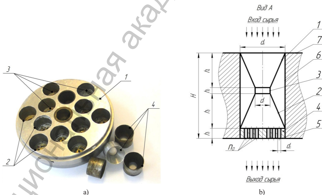
Рис. 2. Общий вид (а) и конструктивная схема (б) матрицы с конфузорно-диффузорными вставками к малому макаронному прессу МИТ-2: 1 – матрица; 2 – колодцы; 3 – вкладыши; 4 – вставки.
