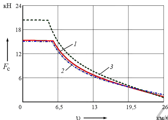
Рис. 4. Зависимость необходимого предварительного статического натяжения от скорости движения трактора в тяговом режиме при включённой подвеске: 1 – Беларусь 1802; 2 – Беларусь 2102; 3 – Беларусь 2103
