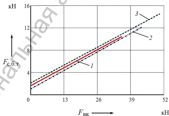
Рис. 3. Зависимость необходимого предварительного статического натяжения от усилия на ведущем колесе трактора с заблокированной подвеской в режиме трогания: 1 – Беларус 1802; 2 – Беларус 2102; 3 – Беларус 2103
