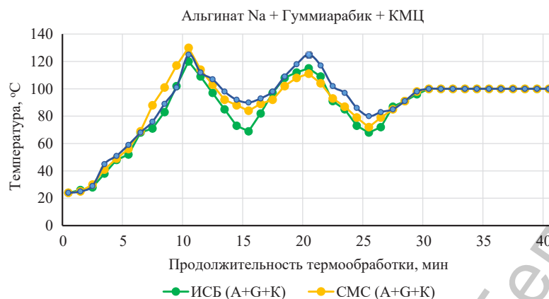
Рис. 2. Изменение температуры в процессе уваривания конфетной массы, приготовленной с использованием БПС, содержащих ИБС и СМС и одинаковую тройную смесь полисахаридов (A + G + K), по сравнению с контролем и в зависимости от продолжительности термообработки
