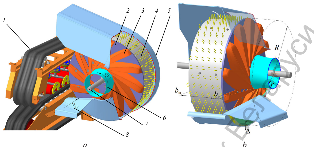
Рис. 1. Конструкция роторного бильно-вычесывающего устройства: a – общий вид устройства ( 1 – зажимной транспортер; 2 – ротор; 3 – бичи; 4 – вычесывающе-транспортирующая щетка; 5 – кожух; 6 – кольцо; 7 – вал ротора; 8 – стол); b – общий вид ротора.
