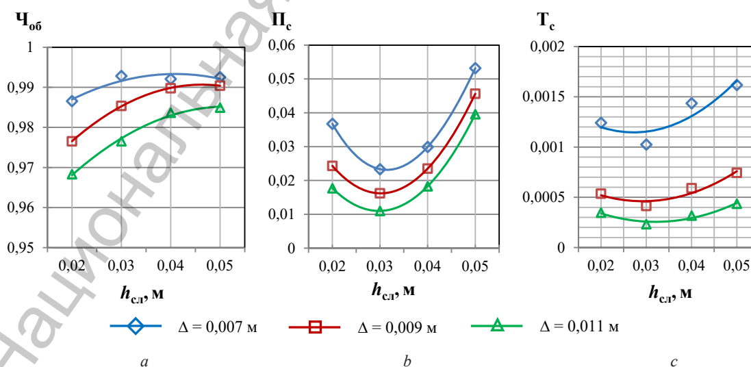
Рис. 4. Графики зависимости чистоты обмолота ( a ), степени повреждения стеблей ( b ) и степени повреждения семян льна ( c ) от толщины ленты льна
