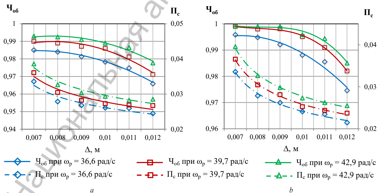
Рис. 6. Зависимости чистоты обмолота и степени повреждения стеблей льна от зазора между ротором и декой в фазе желтой спелости (а) и в фазе бурой спелости льна (b)
