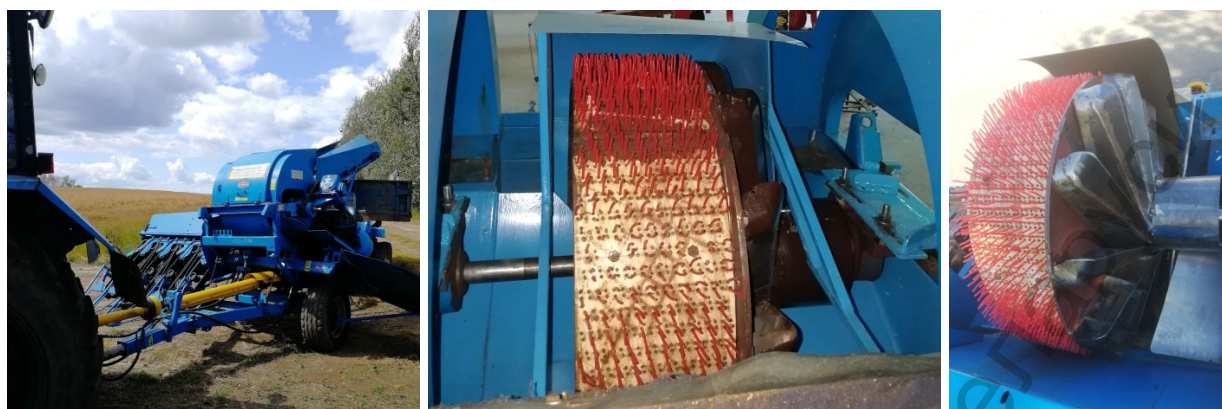
Рис. 2. Льноуборочный комбайн «Двина-4М» с роторным бильно-вычесывающим устройством: а – общий вид МТА; б – обмолачивающее устройство в камере обмолота с кожухом; с – обмолачивающее устройство в камере обмолота без кожуха
