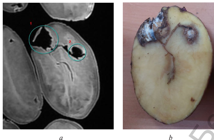
Рис. 5. Результаты сканирования клубней картофеля группы с искусственно созданными повреждениями (a); дефектный клубень картофеля (в разрезе) (b) Fig. 5. Scanning results of potato tubers group with artificially created damages (a), defective potato tuber (in section) (b)
