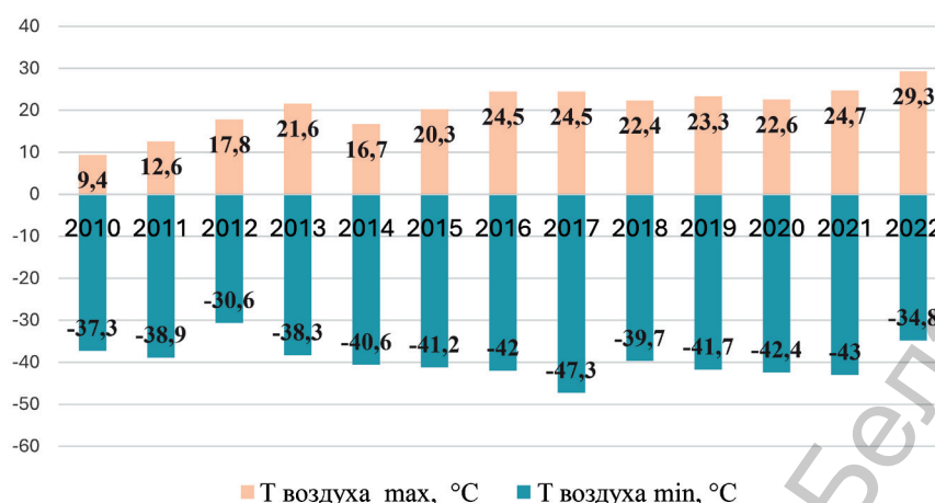
Рис. 5. Многолетнее наблюдение за колебаниями температуры воздуха на полуострове Таймыр, 2010–2022 гг.
