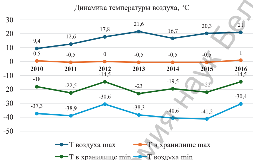
Рис. 1. Наблюдение и регистрация показателей температуры воздуха в хранилище и окружающей среде, мыс Депо, п-ов Таймыр, 2010–2016 гг.
